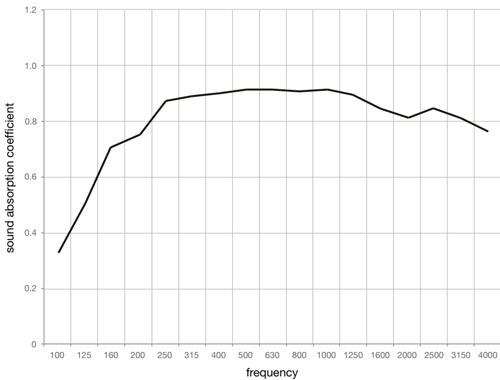
Basalt (NRC 0.90)
